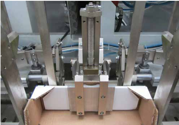
Long and short side doubling Raddoppi testate e fiancate Verdoppelte Kopfseiten und Seitenwände Paredes dobles en las partes superiores y en los laterales
