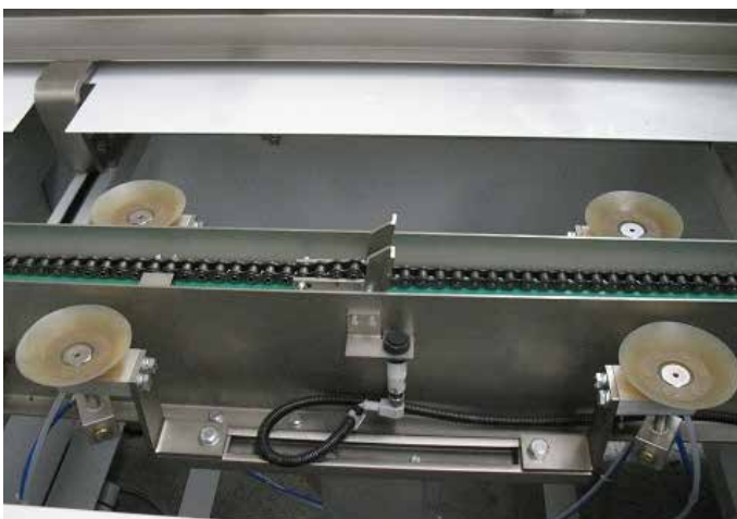
Blanks pick-up Prelievo cartoni Kartonzuschnittes Entnahme Toma de carton
