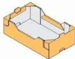
Simple tray with long and short side doubling Vassoio semplice con raddoppio testate e fiancate
