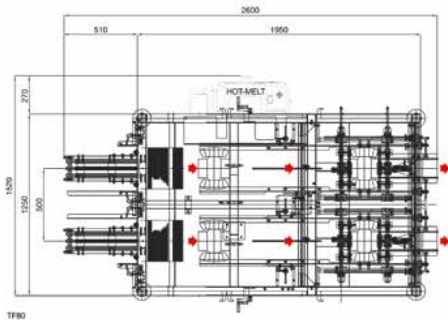
Tray forming zone Zona formatura vassoi Trayaufrichtbereich Zona de formación bandejas
